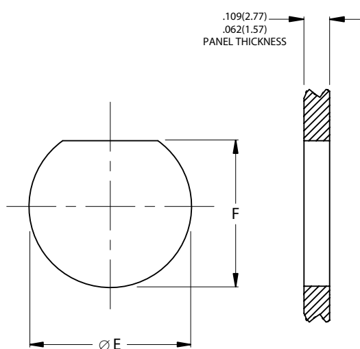
JAM NUT
